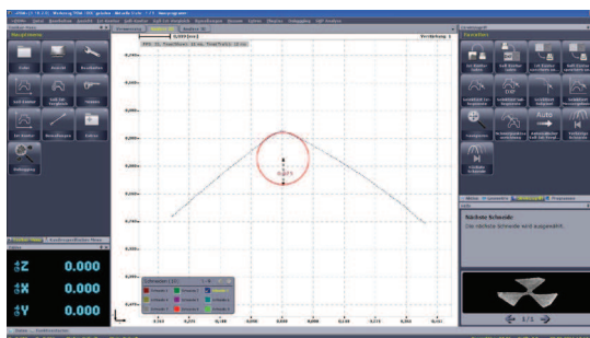
Vyhodnocení rádiusu v řezu
