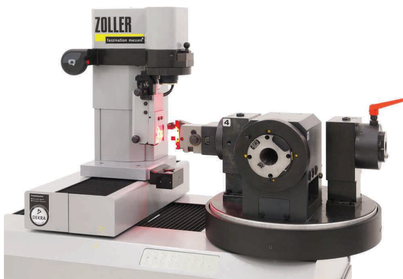
»hyperion 300« s revolverovým stolem \varnothing 450 mm, kamerou pro kontrolu středu osy obrábění a CNC řízeným nastavením optiky.
